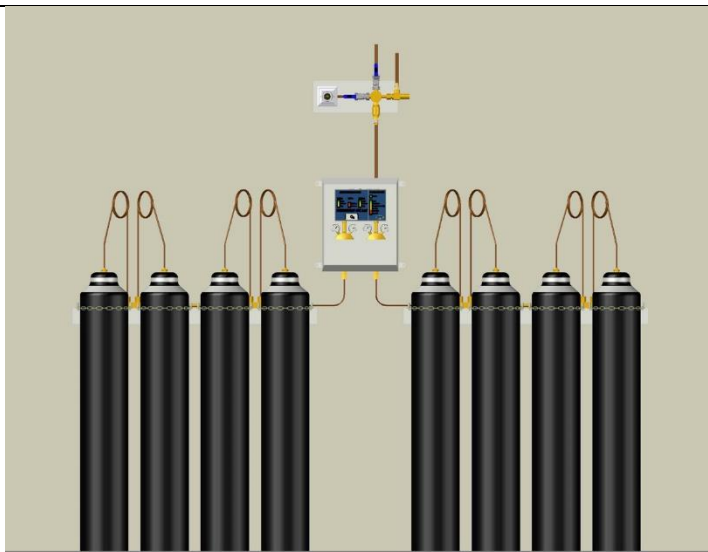
Hộp phân phối khí Hãng sản xuất: Precision (CPX) – Anh
